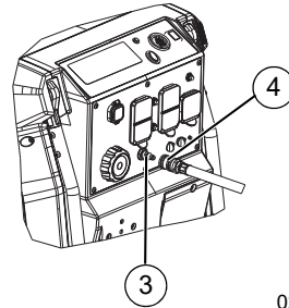
Figure 2-15. Raccorder et débrancher le flexible PL
