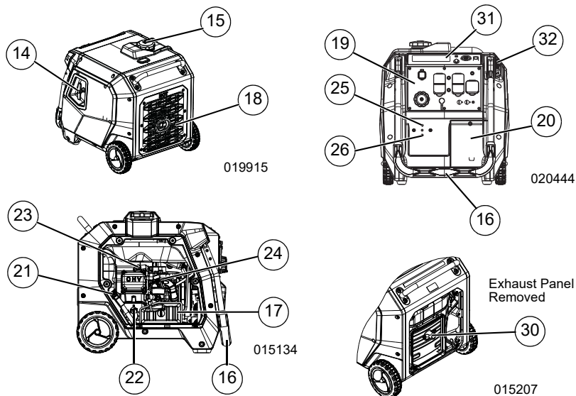
Figura 2-1. Características y controles
