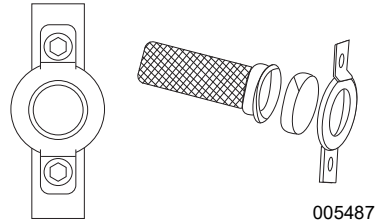
Figure 4-9. Filtre de pare-étincelles
