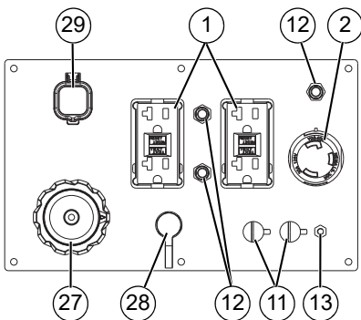
Figure 2-3. Panneau de commande avant
