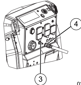
Figura 2-15. Conecte y desconecte la manguera de PL
